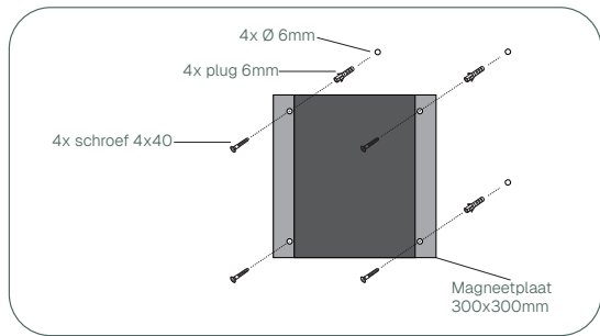
Magneetplaat t.b.v. muurmontage
