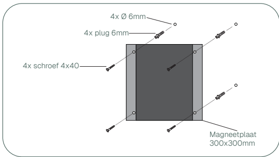
Plaque magnétique pour fixation murale
