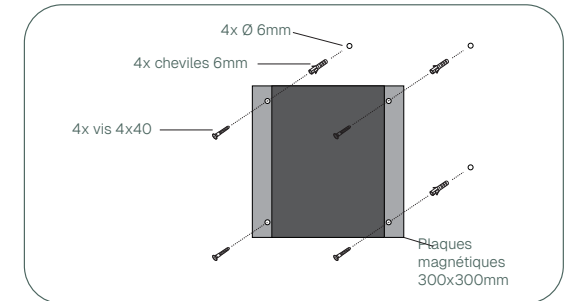
Magnetplatte t.b.v. muurmontage
