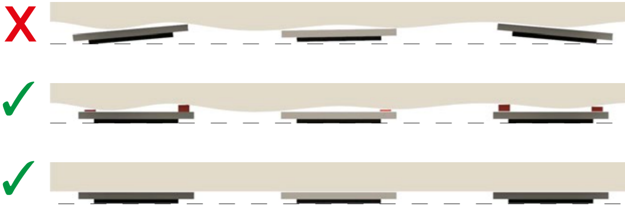
Voorbeeld 1 - Boven-aanzicht -
