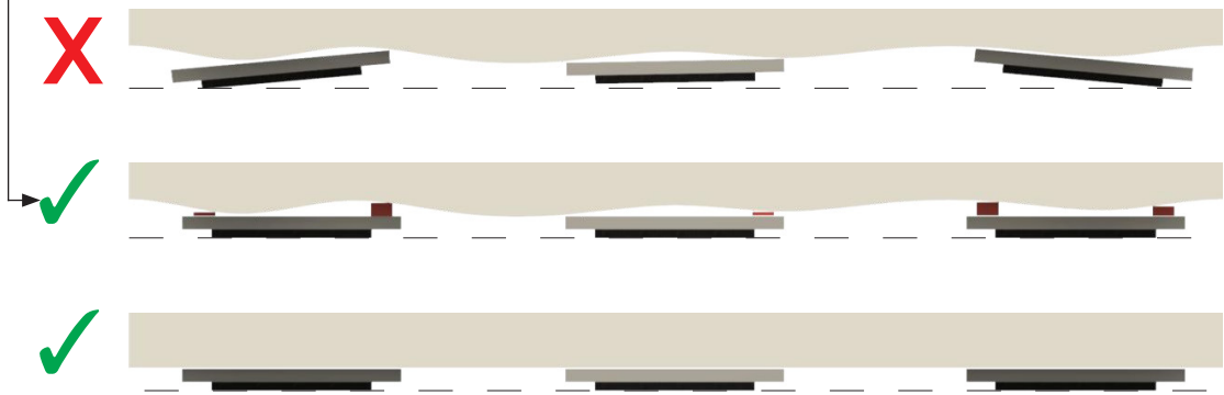
L'esempio 1 - Visto dall'alto -
