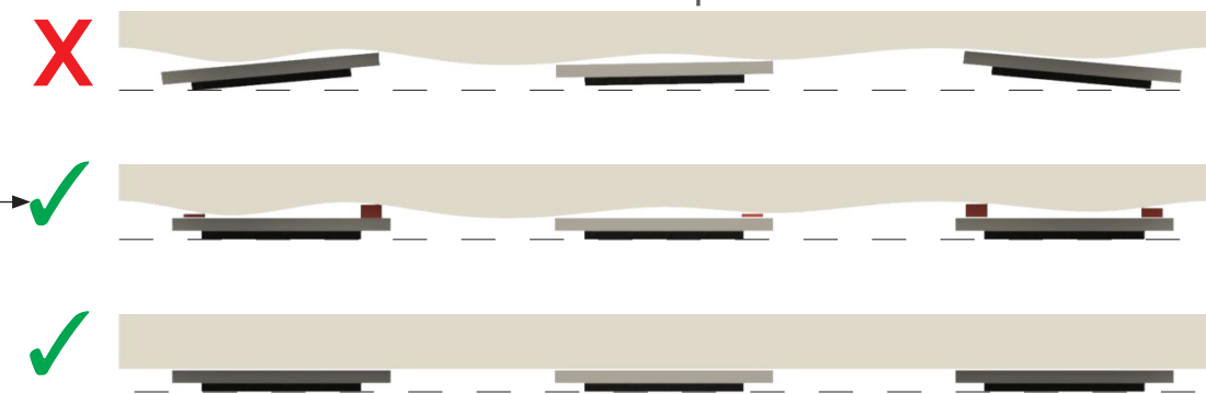
Exemple 1 - Vue en plan -
